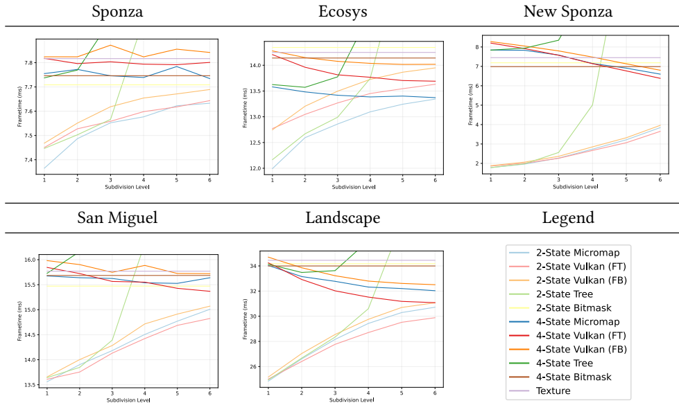
(b) RTX 3080
